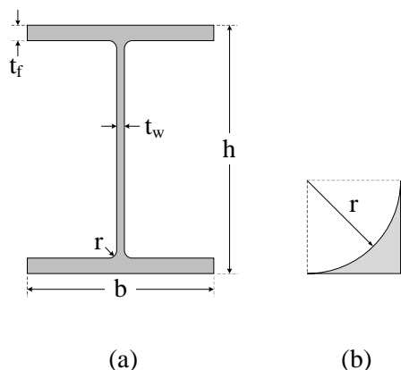
Gambar 2. (a) Bentuk tipikal penampang profil-I canai panas, (b) Bagian sudut pertemuan pelat badan dan pelat sayap.
